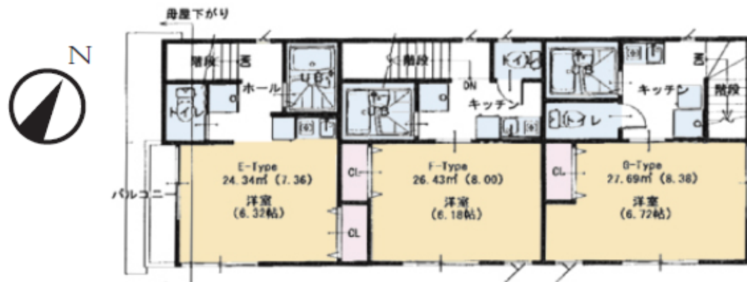
3F平面図
